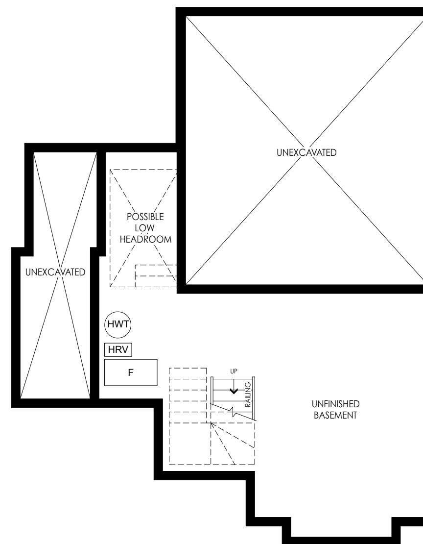
ELEVATION A
